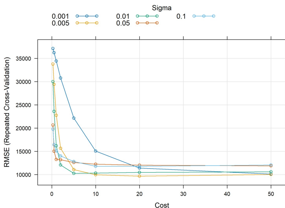
Figura 15: Curva de calibração de hiperparâmetros do modelo SVM (RMSE por validação cruzada repetida).
