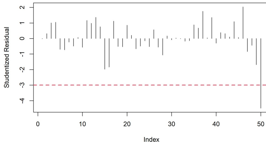
Figura 6: Resíduos estudentizados por observação, com linha de corte em -3 desvios-padrão.
